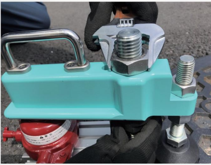
上下のナットでフックを固定する
