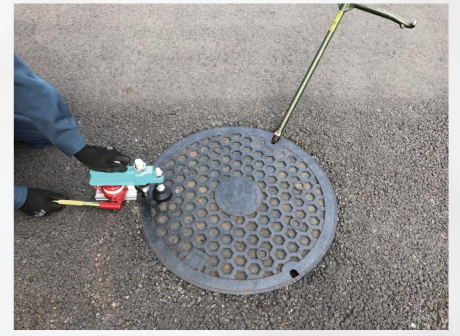
蓋が持ち上がったら ボールを使用して蓋を開ける
